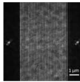
図3: 22nm世代用テストパターンの観察例。白線部がEUVの強度が大きいマスクの開口部を示す。白線の幅は88nmで、露光装置により1/4に縮小焼付けされ、半導体デバイス上で22nm幅の配線パターンとなる。
